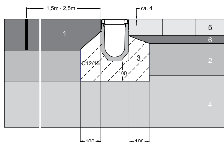
A15 betongblock eller stenbeläggning
