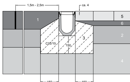
B125 betongblock eller stenbeläggning
