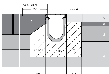
C250 betongblock eller stenbeläggning
