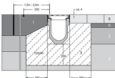
D400, E600 betongblock eller stenbeläggning
