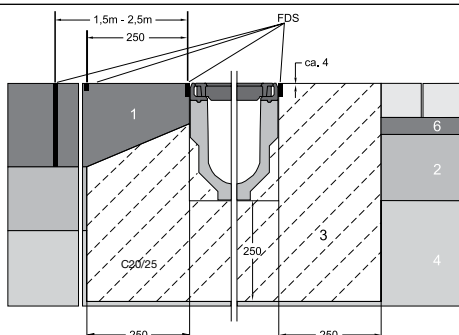
F900 betongblock eller stenbeläggning
